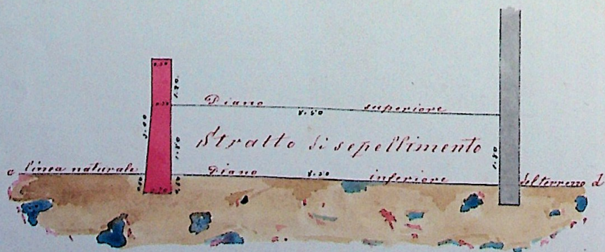
Sezione c-d (Par. I fig. 1°) (figura 9°)
